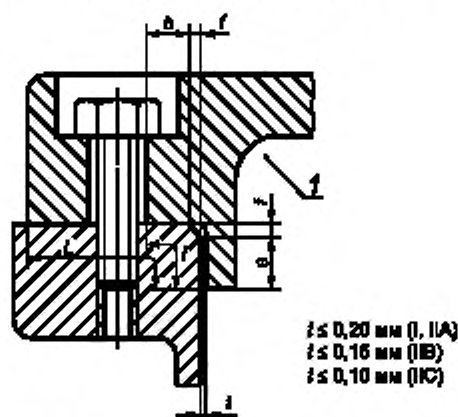
Рисунок 6 — Отверстия на поверхностях плоскоцилиндрических соединений (пример 1)
