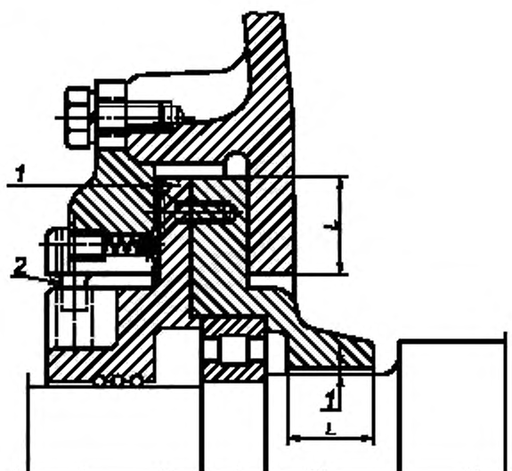
Рисунок 19 — Соединение с плавающими втулками для валов вращающихся электрических машин
