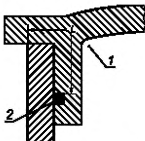
Рисунок 10 — Иллюстрация требований к прокладкам (пример 1)
