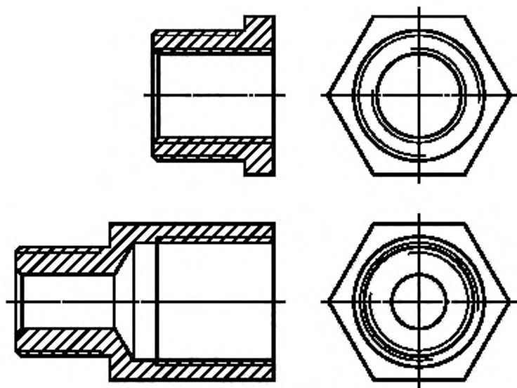
Рисунок С.3 — Примеры резьбовых Ex-переходников
