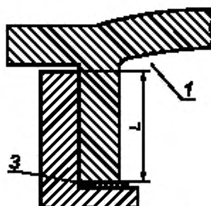
Рисунок 12 — Иллюстрация требований к прокладкам (пример 3)
