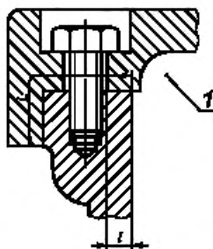
Рисунок 7 — Отверстия на поверхностях плоскоцилиндрических соединений (пример 2)
