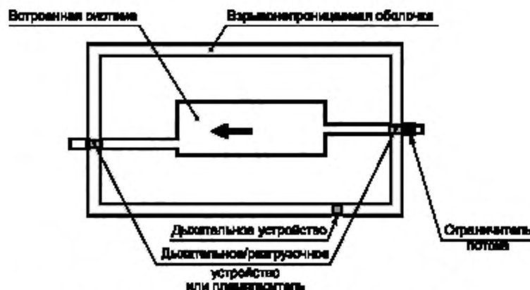
Рисунок G.1 — Взрывонепроницаемая оболочка со встроенной системой
