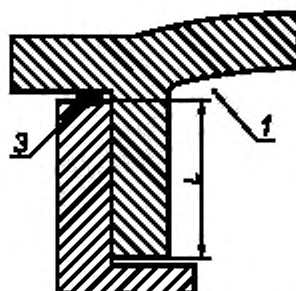
Рисунок 13 — Иллюстрация требований к прокладкам (пример 4)
