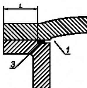
Рисунок 15 — Иллюстрация требований к прокладкам (пример 6)
