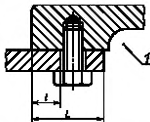
Рисунок 4 — Отверстия на поверхностях плоских соединений (пример 2)
