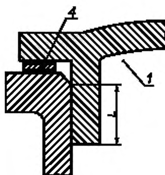
Рисунок 15 — Иллюстрация требований к прокладкам (пример 6)
