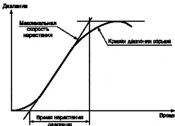
Рисунок 23 — Пример кривой правильной формы
