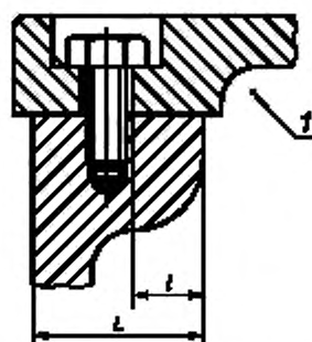
Рисунок 5 — Отверстия на поверхностях плоских соединений (пример 3)
