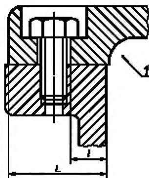
Рисунок 3 — Отверстия на поверхностях плоских соединений (пример 1)
