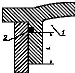
Рисунок 11 — Иллюстрация требований к прокладкам (пример 2)
