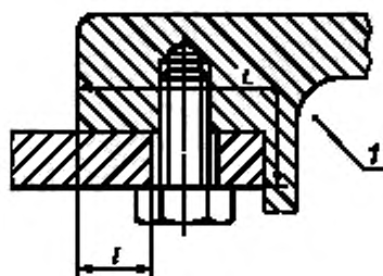
Рисунок 8 — Отверстия на поверхностях плоскоцилиндрических соединений (пример 3)
