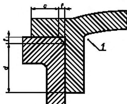
Рисунок 2а — Цилиндрическая часть и плоская часть
