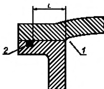
Рисунок 14 — Иллюстрация требований к прокладкам (пример 5)
