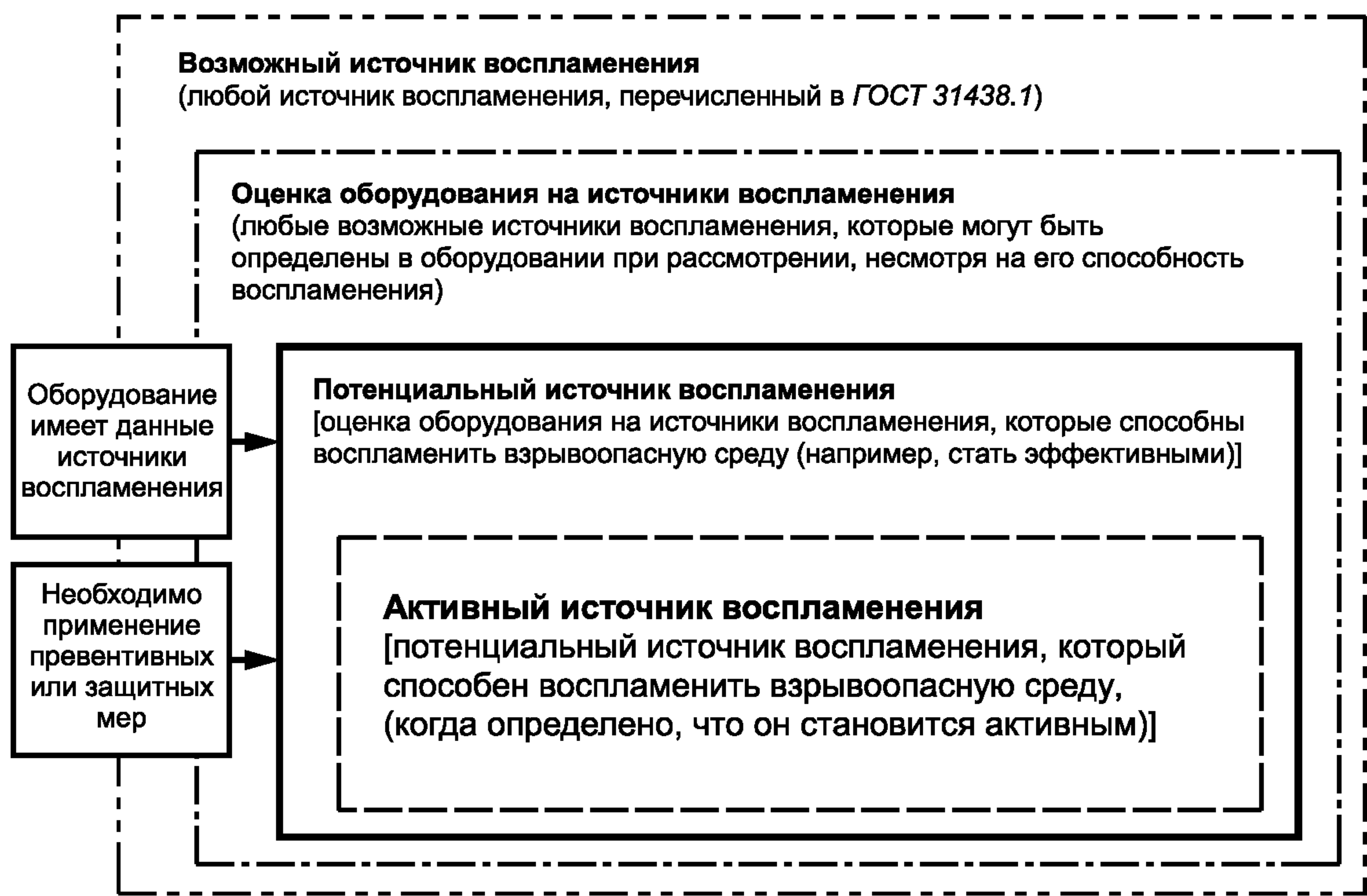
Рисунок А.1 — Соотношение между определениями источников воспламенения
