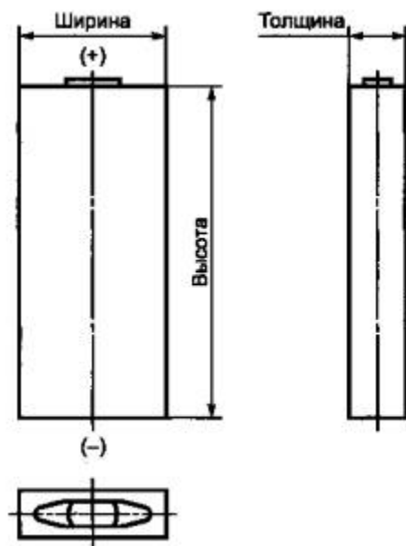
Рисунок 4 - Малогабаритный призматический аккумулятор в чехле
